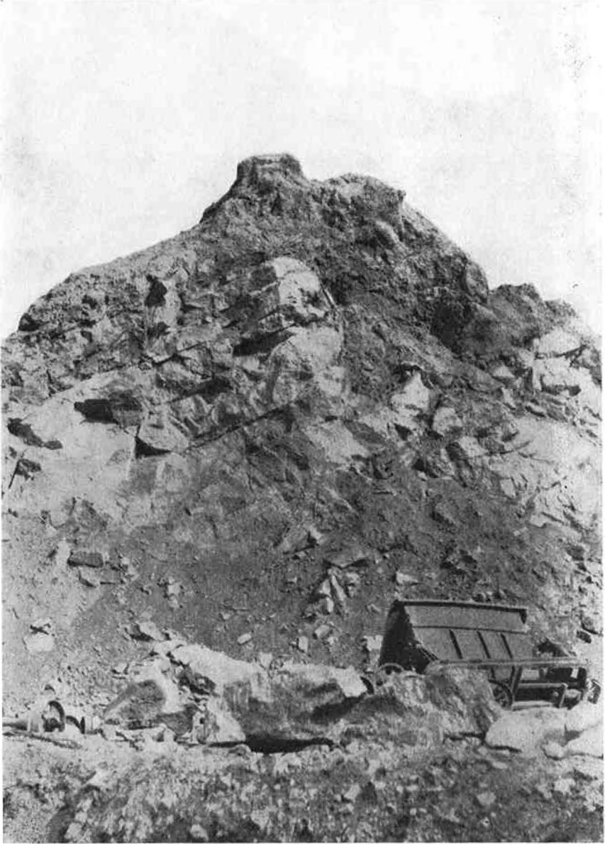
Abb. 5: Nicht abgebaute Ockerpartien im Karstschlot des Magnesit-Tagbaues.
